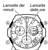
Lancetta delle 24 ore Posizione iniziale corretta della lancetta delle 24 ore e della lancetta dei minuti
