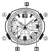
Impostazione del giorno del mese
